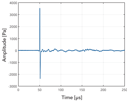
热声发射器的脉冲响应
