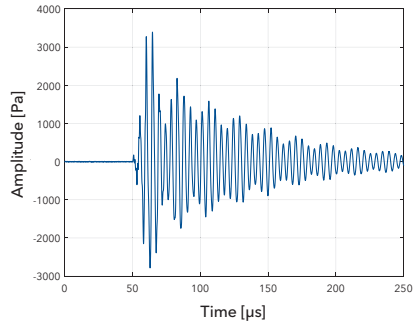
压电发射器的脉冲响应
