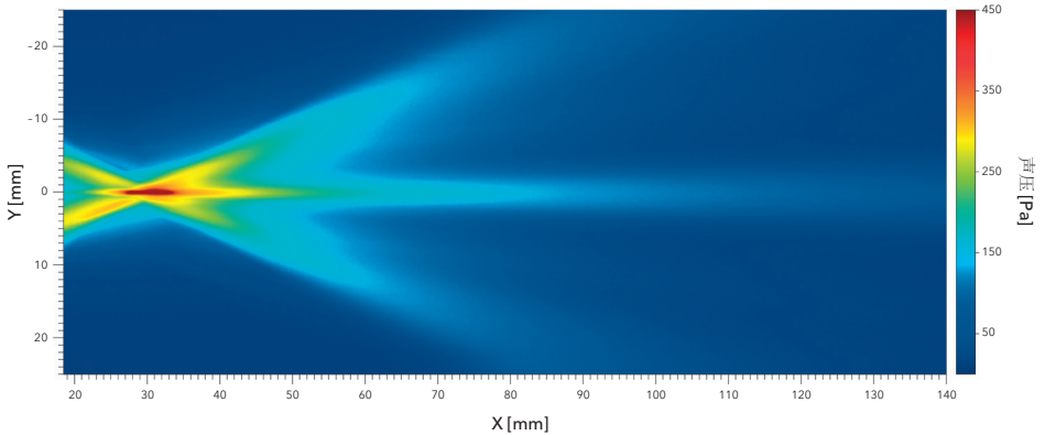
用光学麦克风测量的热声发射器的声场
